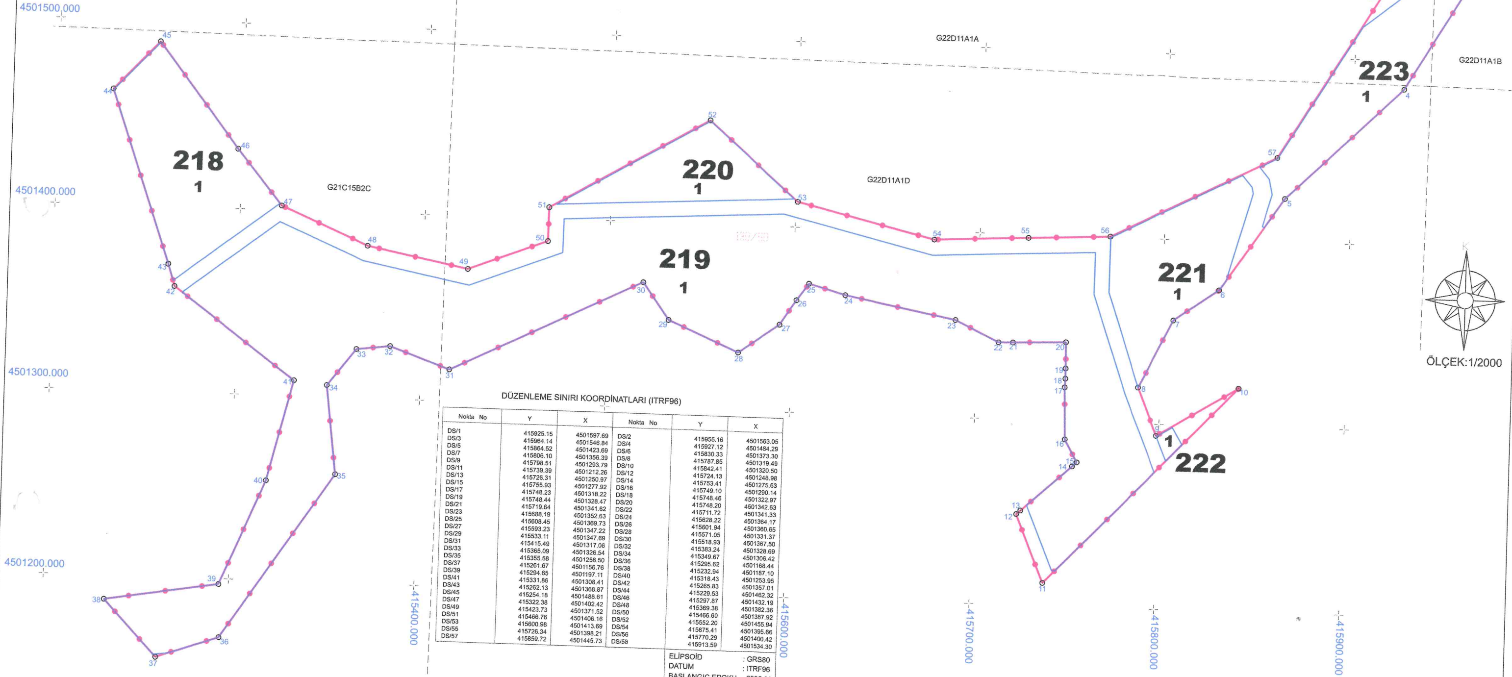
DÜZENLEME SINIRI ALAN HESABI
